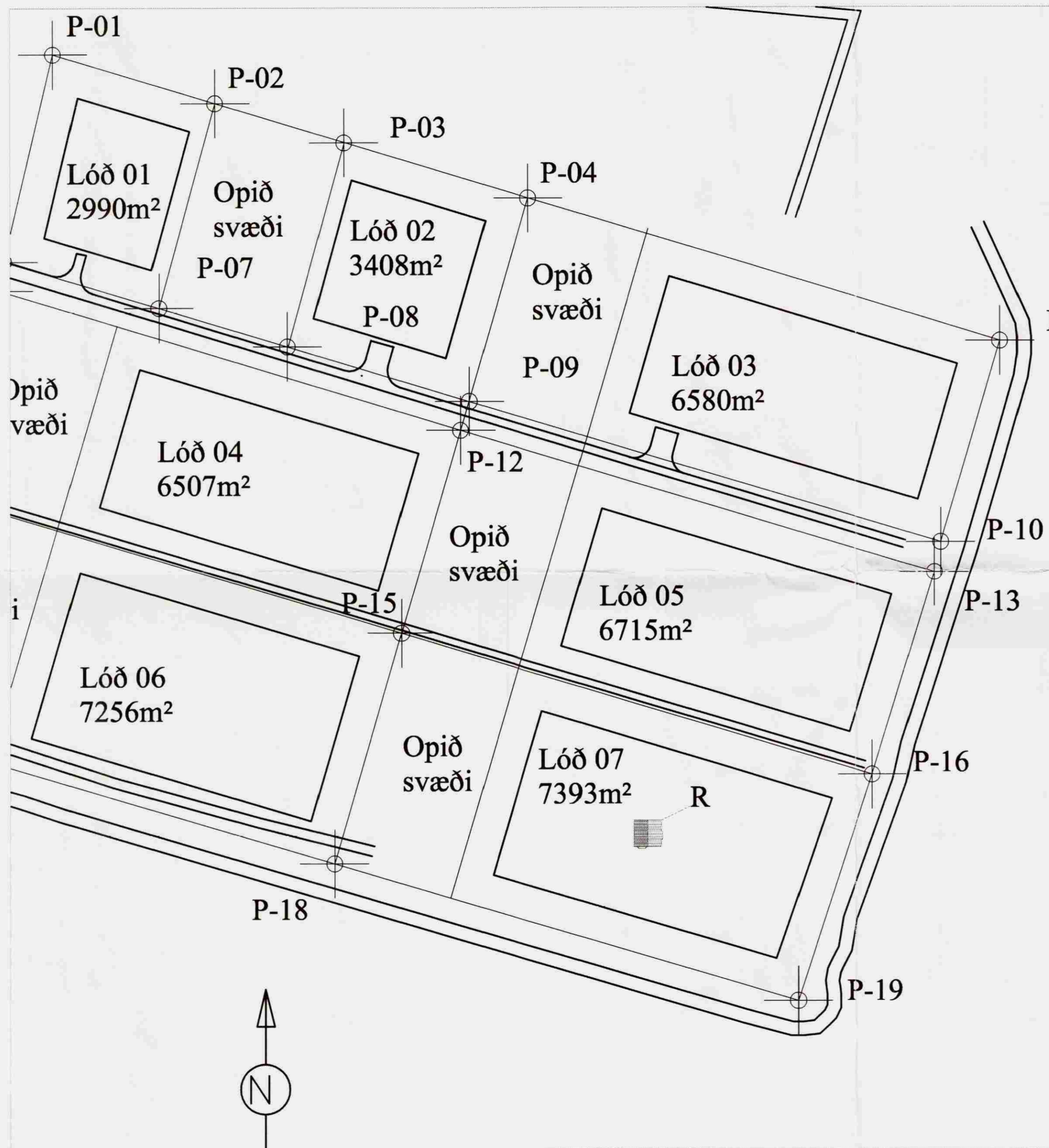
Afstöðumynd 1:1000
