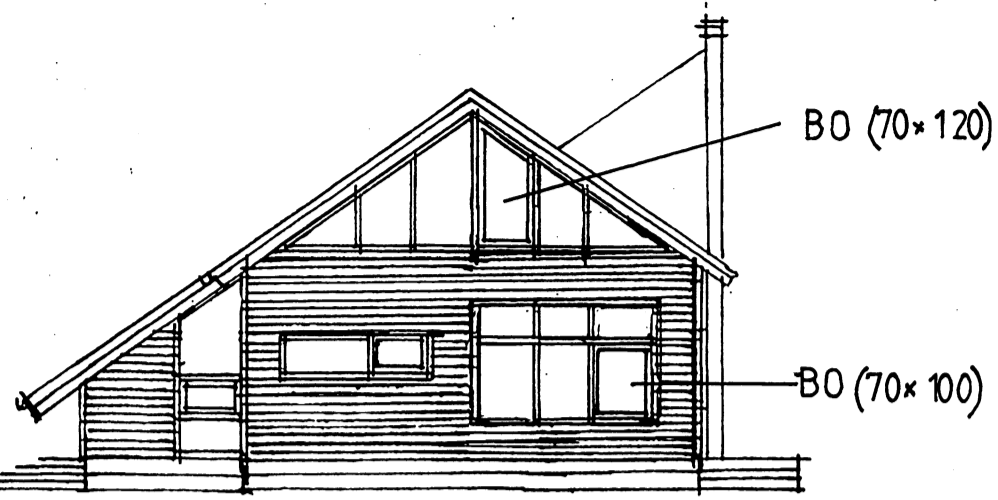
ÚTLIT NORÐUR
