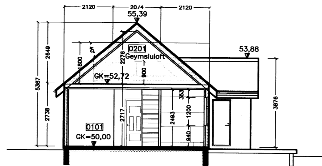
SNID A-A MKV.2
