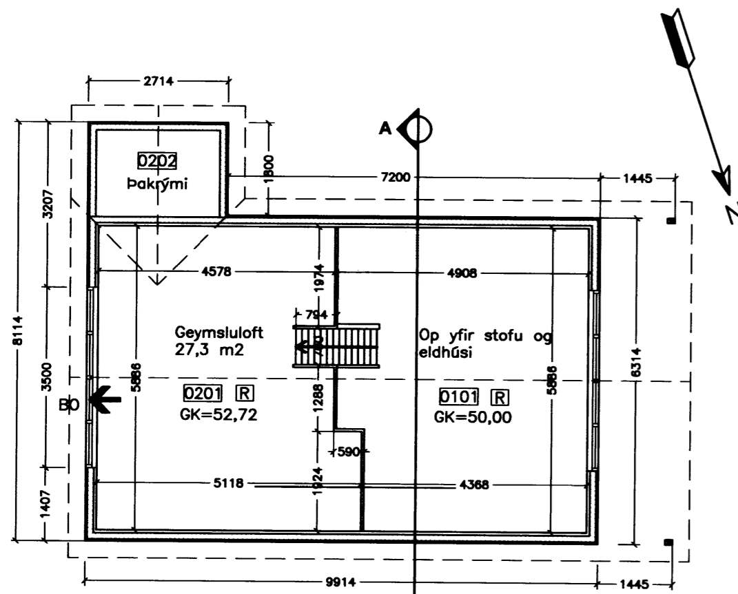
GRUNNMYND 2. HÆÐ MKV.2
