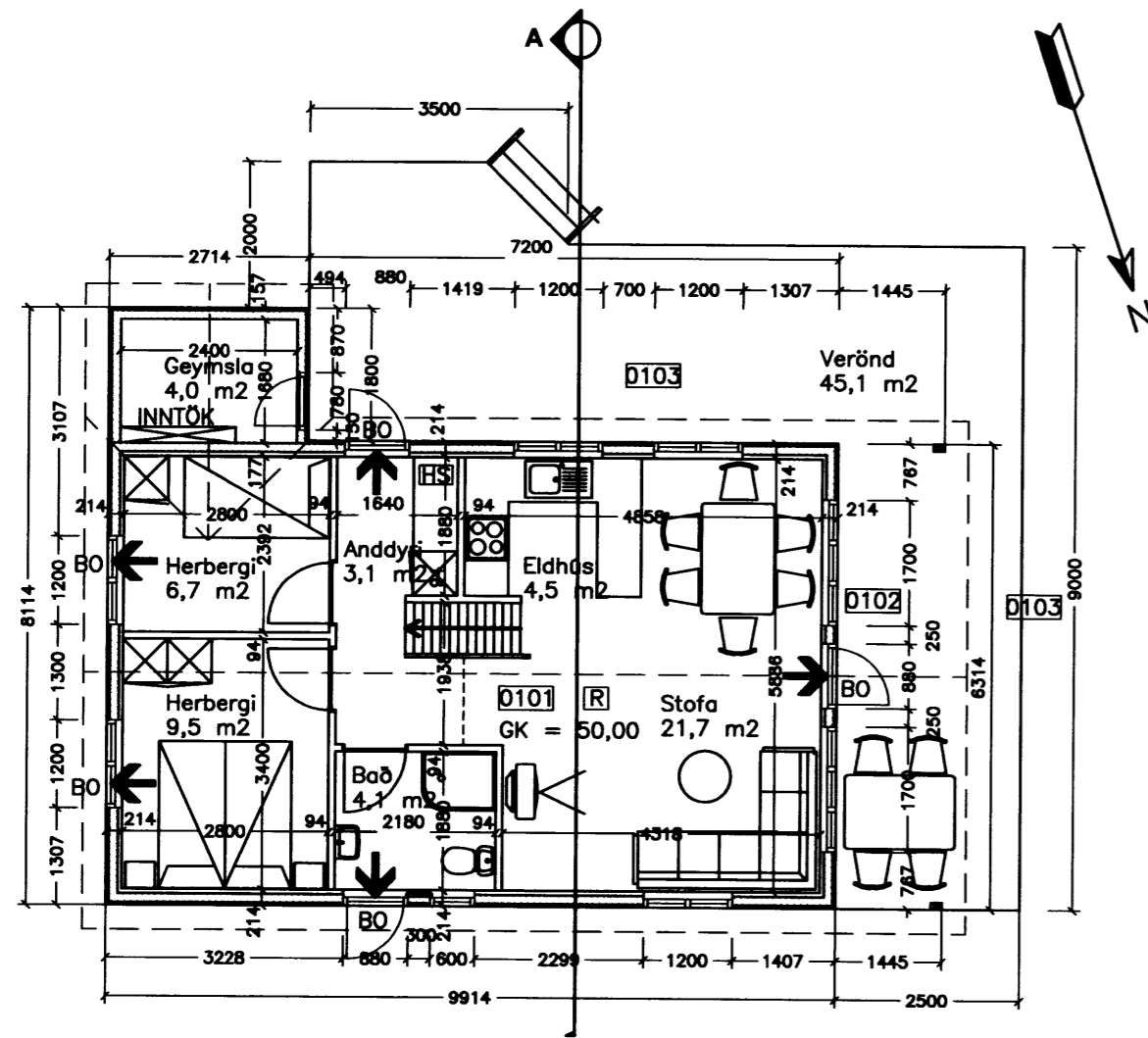
GRUNNMYND 1. HÆÐ MKV.2
