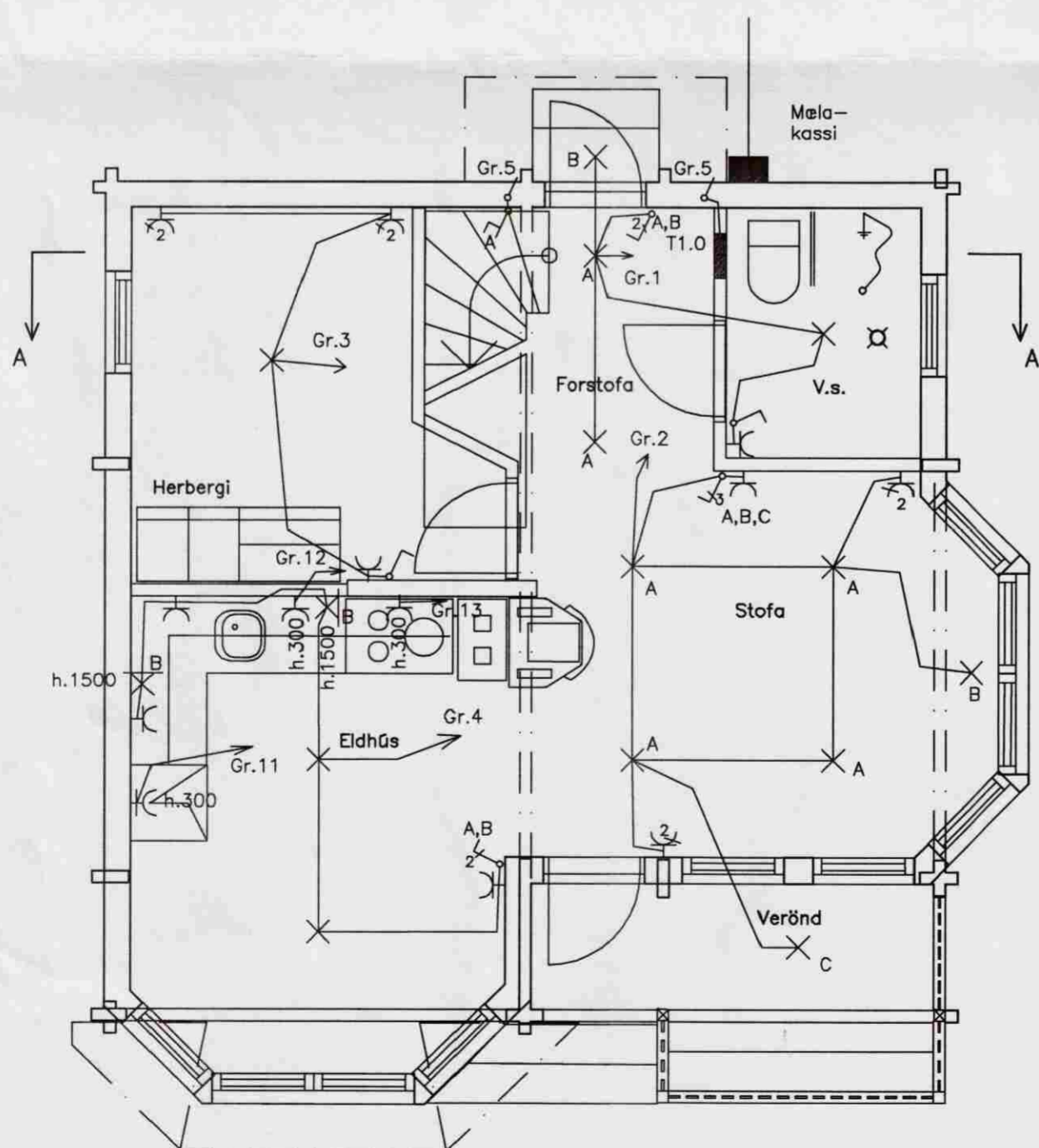
Raflögn mkv. 1:50
