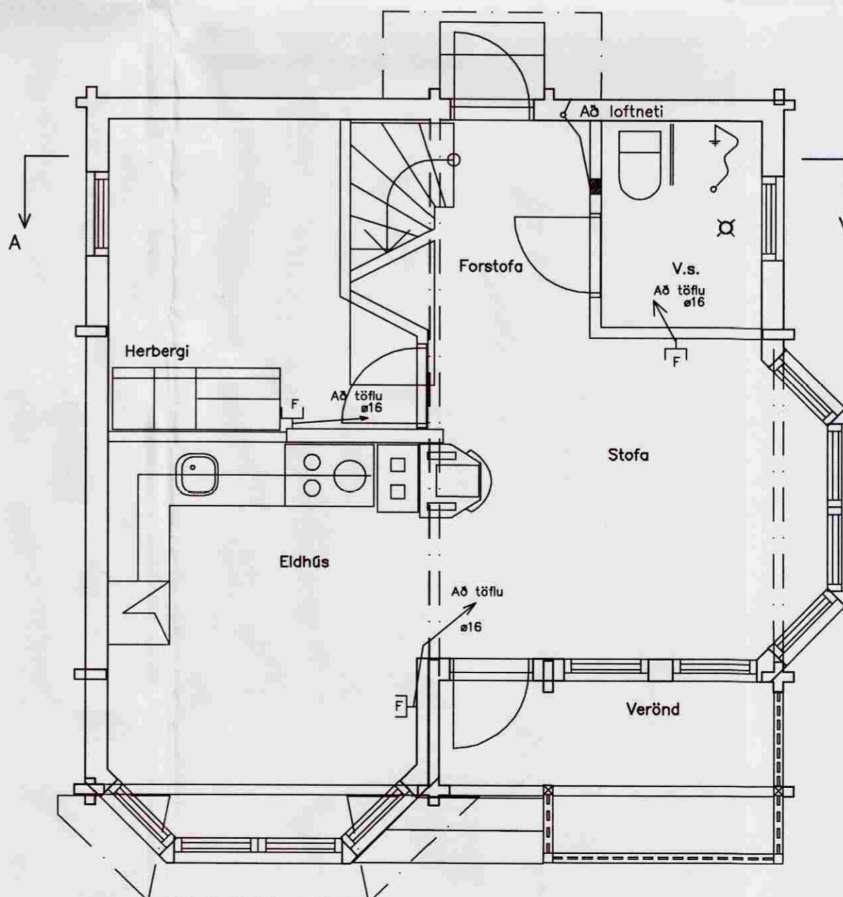
Smáspenna mkv. 1:50
