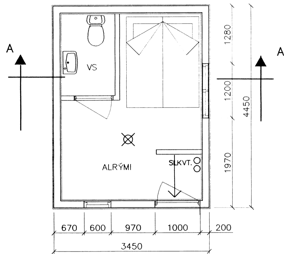
GRUNNMYND 1:50
