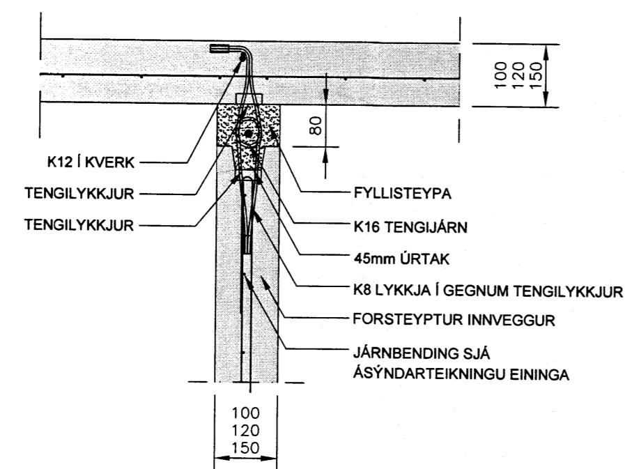
6 SAMSETNING INNVEGGJA 1:10
